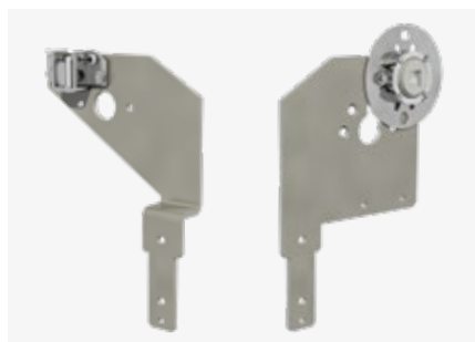
Supports coudés et plats pour actionnement par sangle et chaînette
