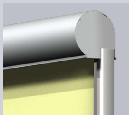
Box (caisson) avec guidage coulisses
