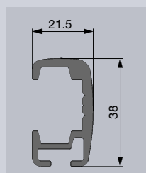
Profil en C arrondi
