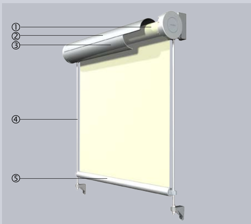
Sigara® Box avec guidage par tiges
